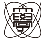
▲電気通信大学の校章。リサージュ図形とは、互いに直角方向に振動する二つの単振動を合成して得られる平面図形のこと。
